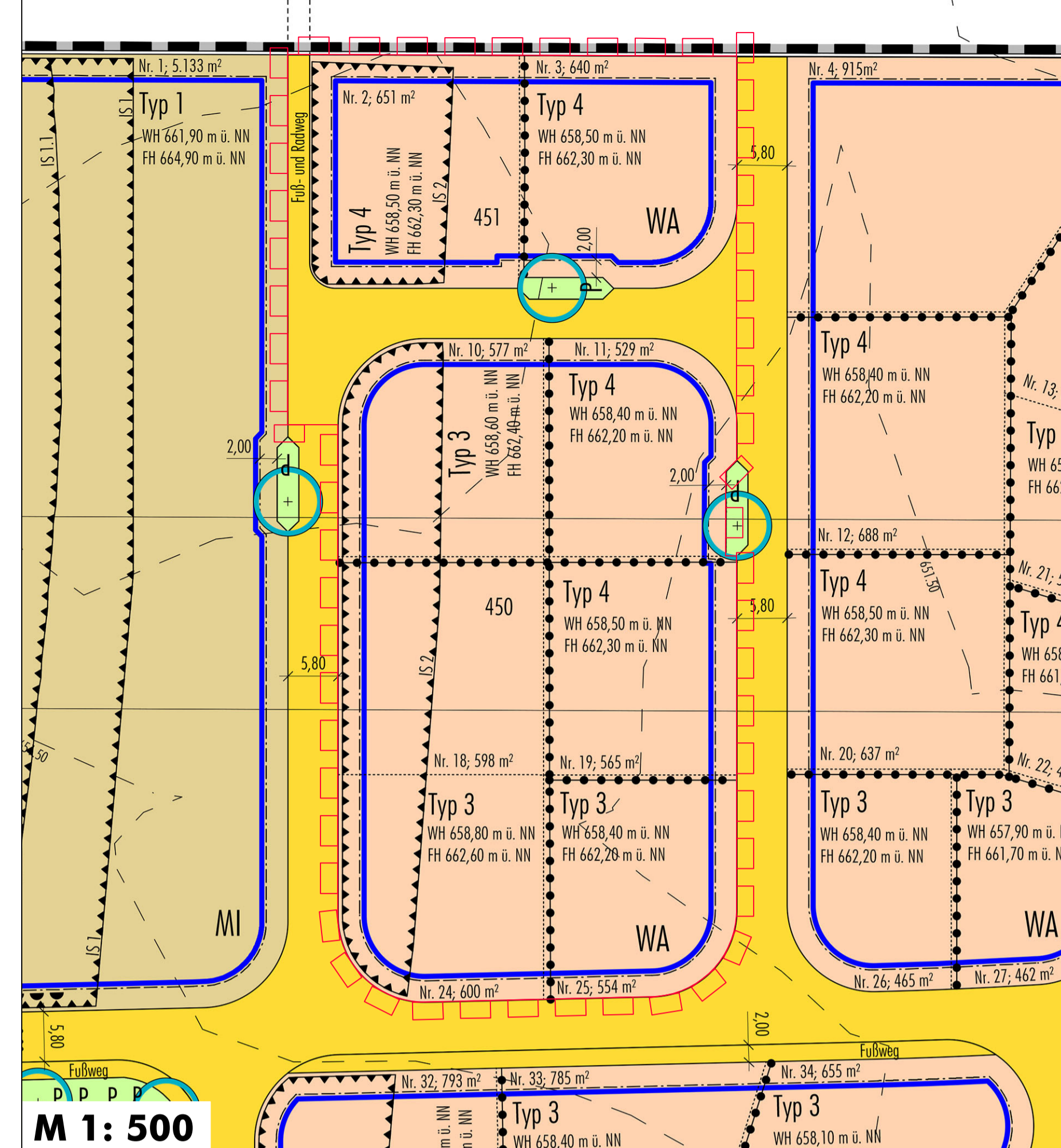
M 1: 500 Bebauungsplan "Becherhalde BA II" (Fassung vom 30.10.2015)
